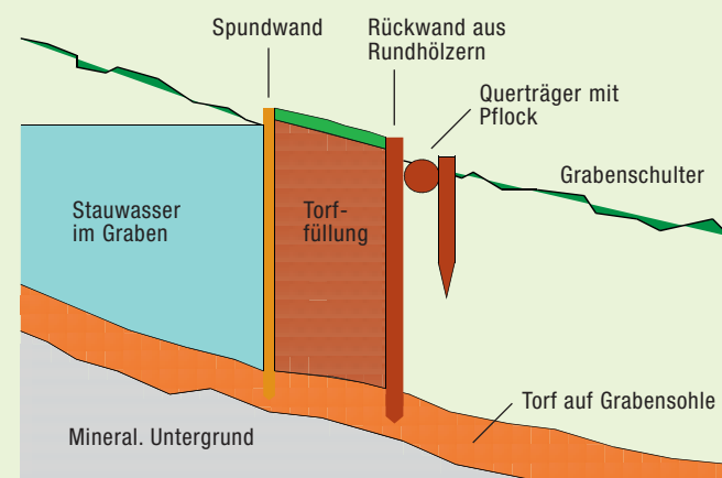
Schematischer Aufbau eines Stauwehres
